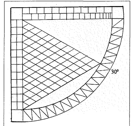
İbnü's-Şâtir'in er-rub'u't-tâmı
